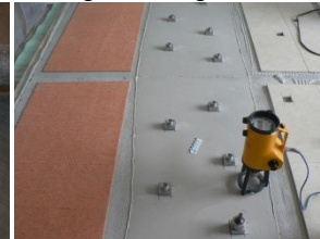
Prüfung Haftzugfestigkeit
